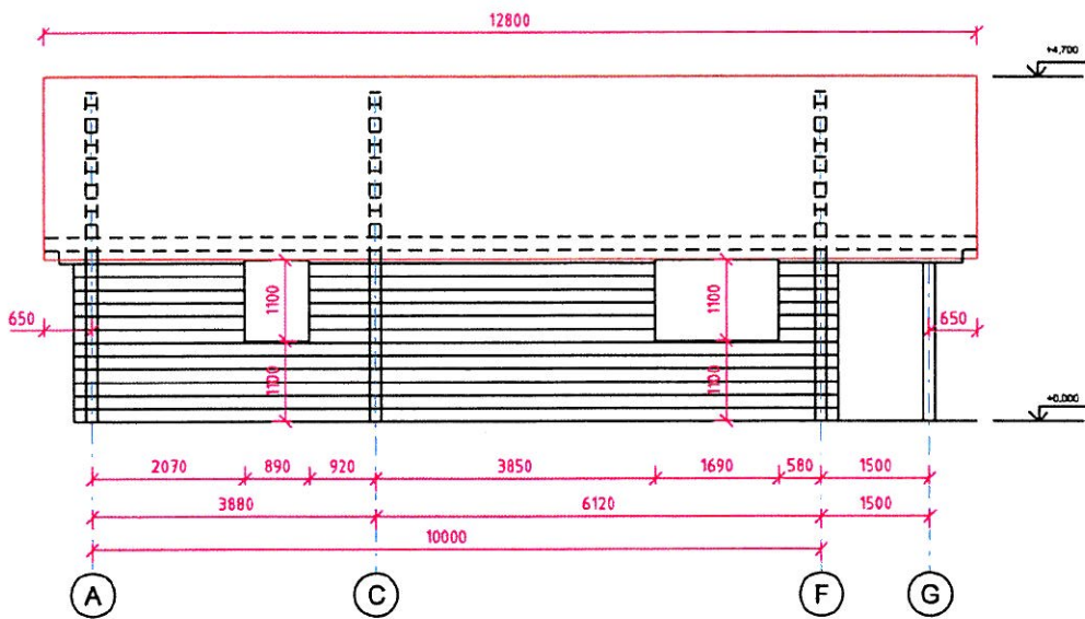
Fasade 3
