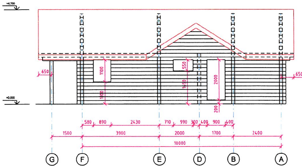
Fasade 1
