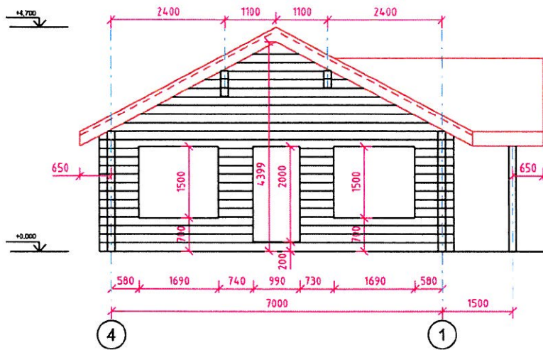
Fasade 2
