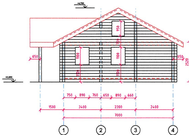
Fasade 4
